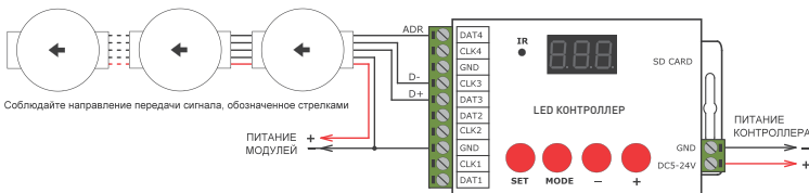
Рис. 2. Подключение DMX-модулей или лент с остальными поддерживаемыми микросхемами
