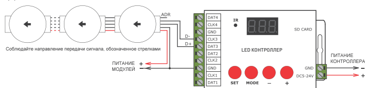
Рис. 1. Подключение DMX-модулей или лент с микросхемами UCS512, TM512AC4
