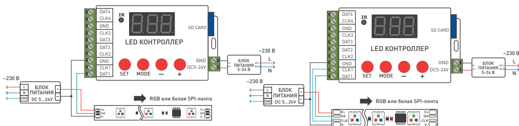
Рис. 1. Подключение SPI-лент к контроллеру
