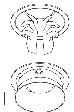
Рис. 3. Демонтаж светильника
