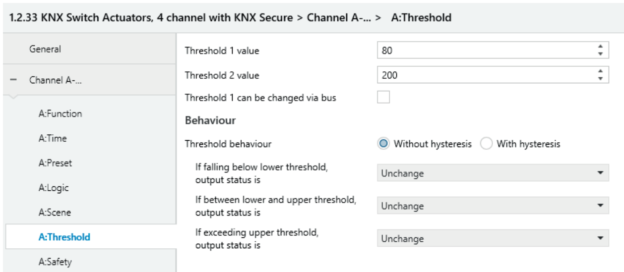
Fig. 4.4.5 Parameter window “X: Threshold”
