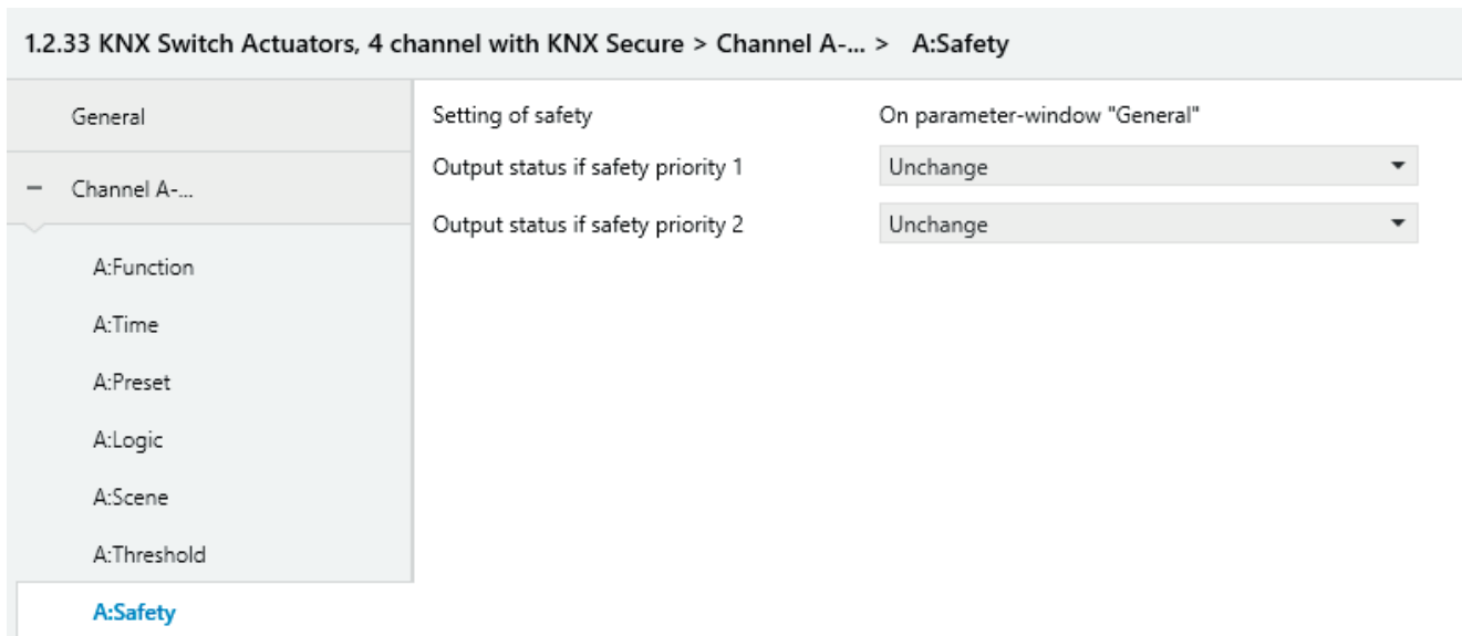
Fig. 4.4.6 Parameter window “X: Safety
