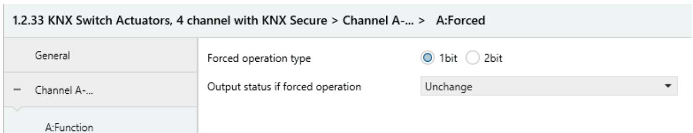
Fig. 4.4.7 Parameter window “X: Forced”
