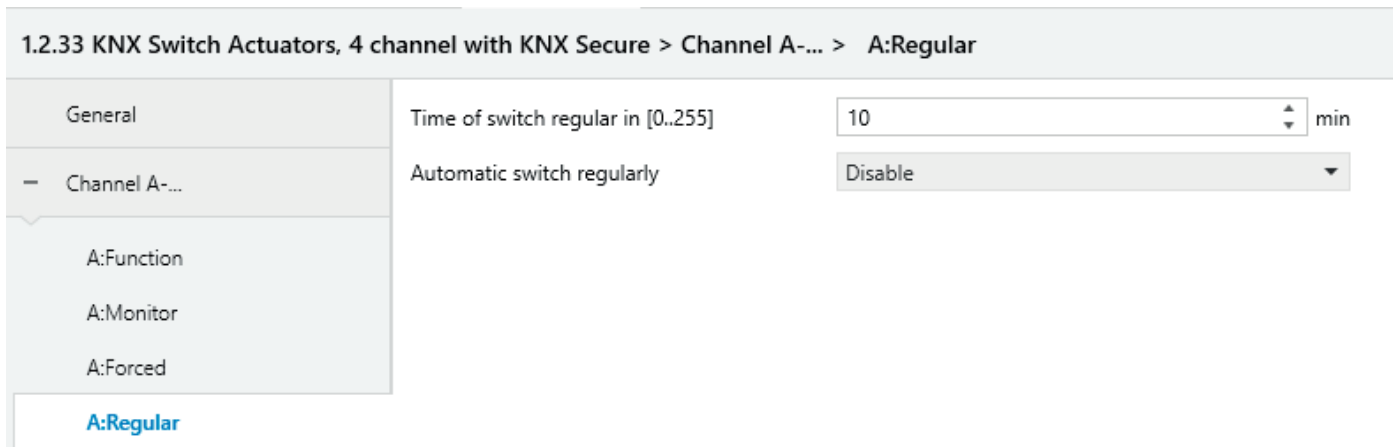
Fig. 4.5.3 Parameter window “X: Regular”
