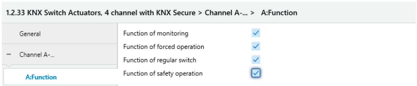
Fig. 4.5(2) Parameter window “X: Function”
