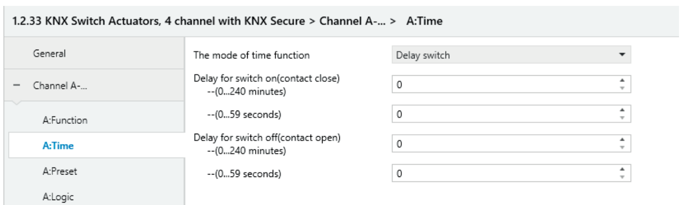
Fig. 4.4.1.1 Parameter window “X: Time”-Delay
