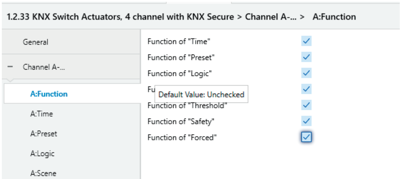
Fig. 4.4(2) Starting parameter window “X: Function”
