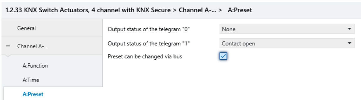
Fig. 4.4.2 Parameter window “X: Preset”
