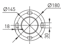
Рис. 2. Чертеж и габаритные размеры фланца OXOR-OT1-D108
