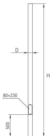
Рис. 1. Чертеж и габаритные размеры опоры OXOR-OT1-D108
