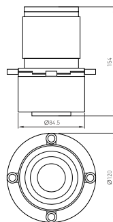
Рис. 1. Чертеж и габаритные размеры
