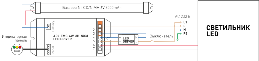
Рис. 3. Схема подключения светильника
